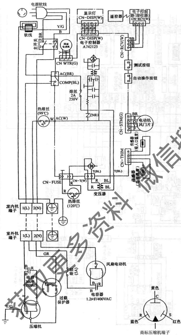
图 15 松下 CS-C95KW、CU-C125KW、CU-C145KW、CS-C145KW 空调器控制电路图
