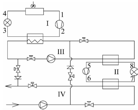
I 空气/水热泵 II 水/水热泵 III 中间水回路 IV 热媒循环回路 图2 单、双级耦合热泵系统图
