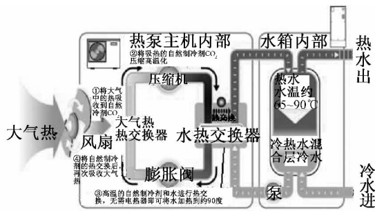
图6 二氧化碳热泵热水器原理图
