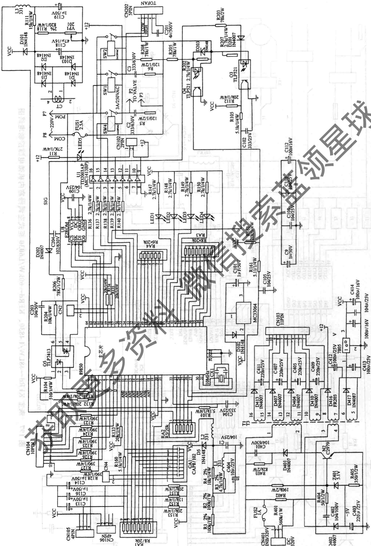
图 196 森宝 KFR—50LW/BP 变频柜式空调器室外机微电脑控制电路图
