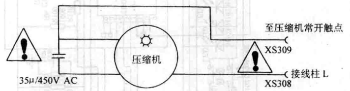
图 207 新科 KFR—35GW/EF1 型绿色空调器室外机控制电路图
