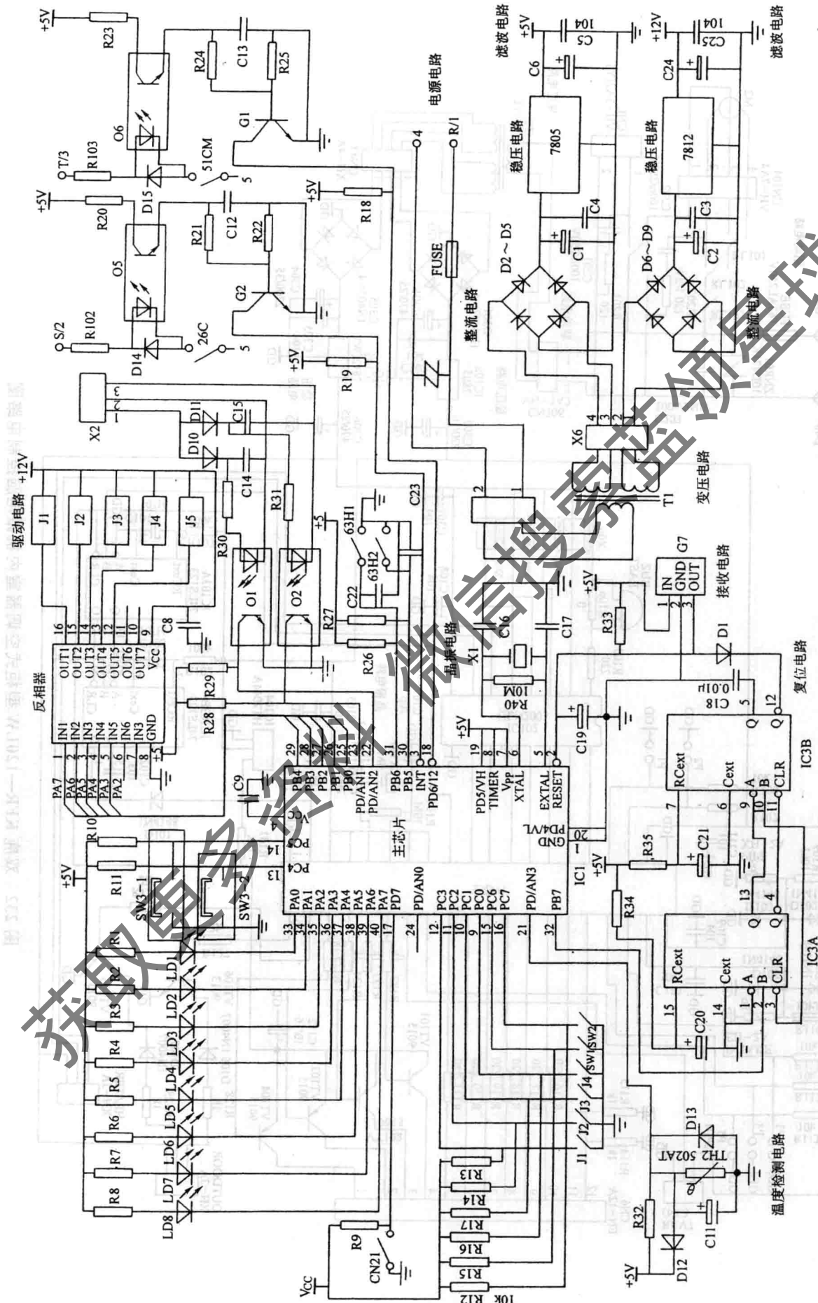
图 233 双鹿 KFR-120LW 型柜式空调器室外机微电脑控制电路图
