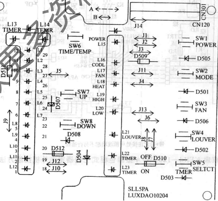
图 229 双鹿 KFRd—120LW/A 型柜式空调器室内机显示板控制电路图
