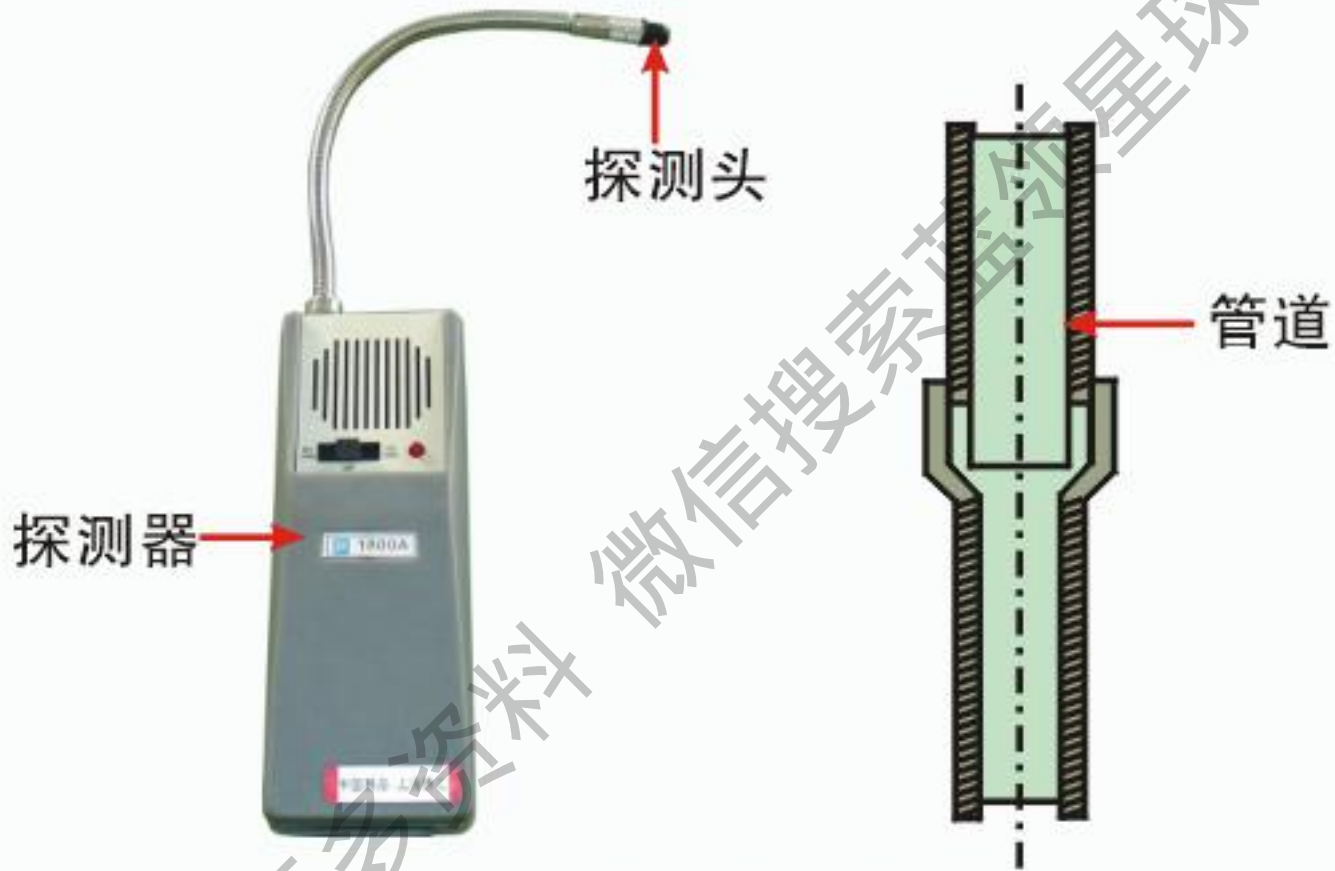
(a) 检漏仪外形
