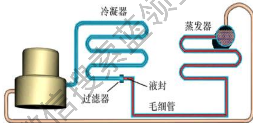
(a) 毛细管阻力恰当
