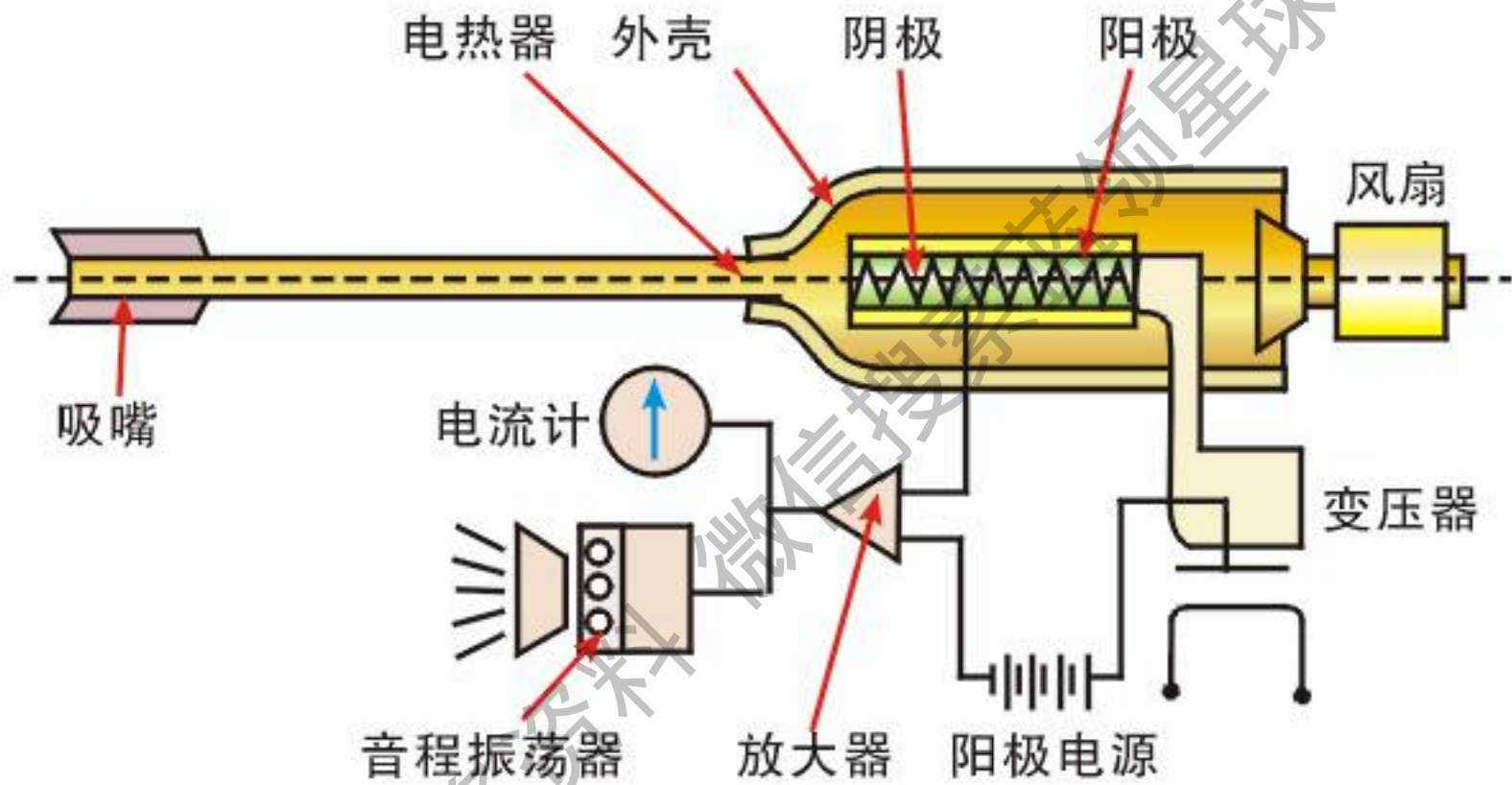
(b) 检漏仪结构
