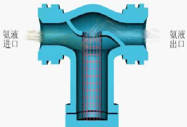
氨液过滤器
