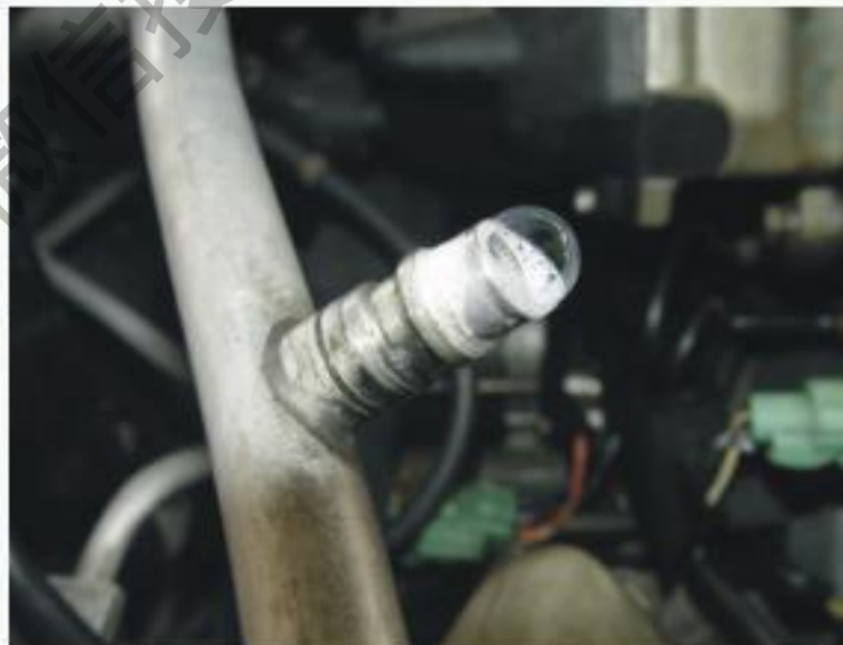
肥皂液检漏法
