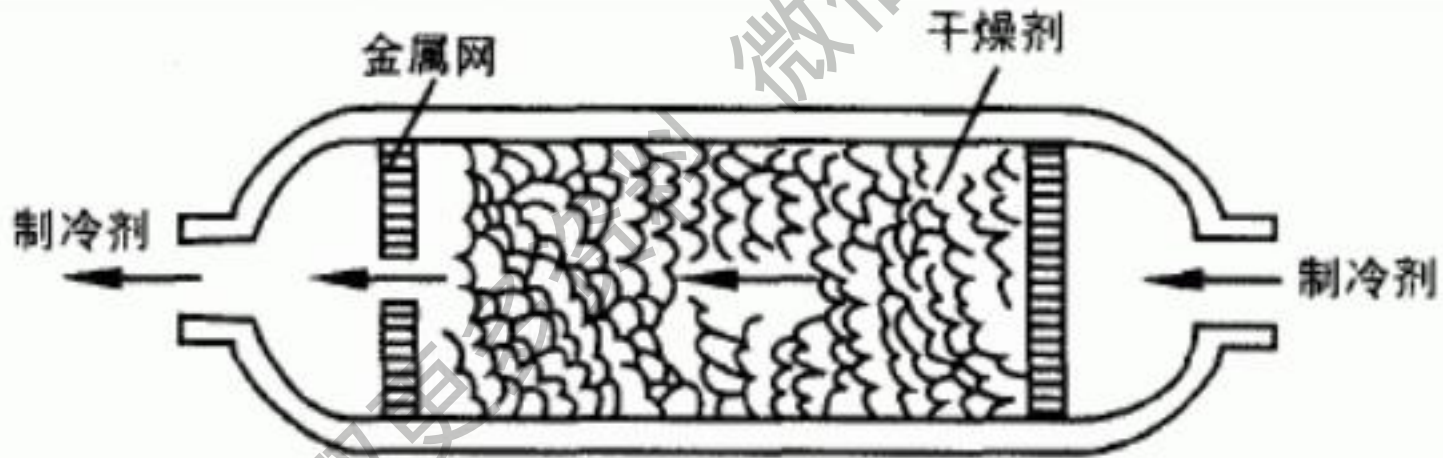
图 1 干燥过滤器的结构图
