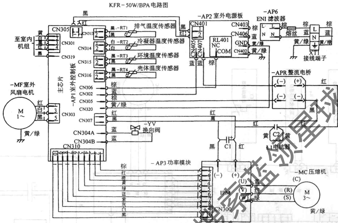
图 126 春兰 KFR-50LW/BPA 型变频空调器室外机控制电路图
