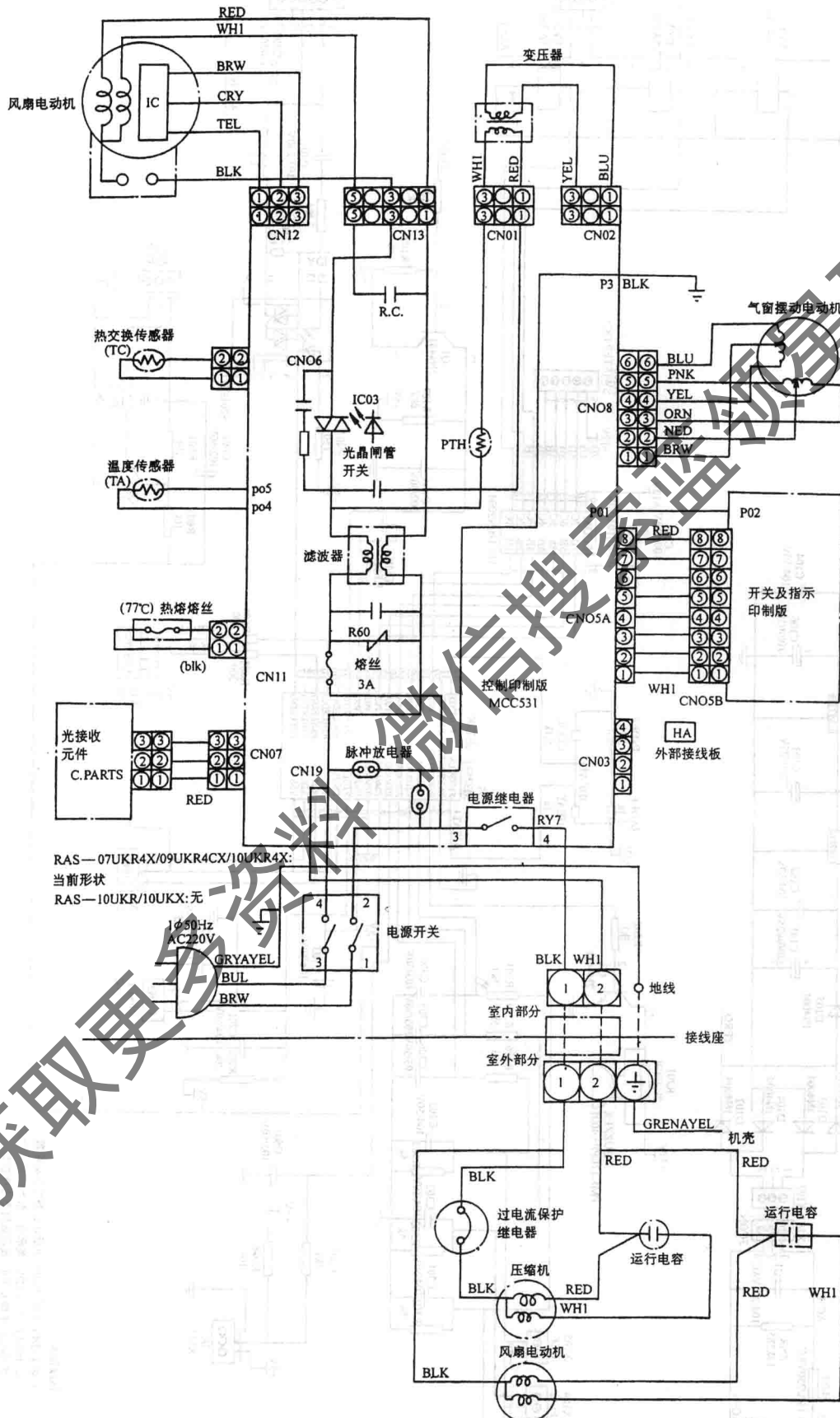
图 35 东芝 RAS—07UKR4X/09UKR4CX/10KR4X、RAS—10NKX/10NAX、RAS—10NK4X/10NA4X 空调器控制电路图
