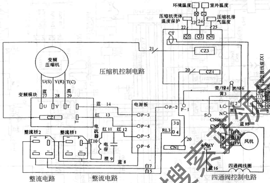
图 23 美的 KFR—50LW/FBPY 变频空调器室外机控制电路图
