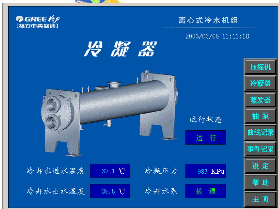
冷凝器界面
