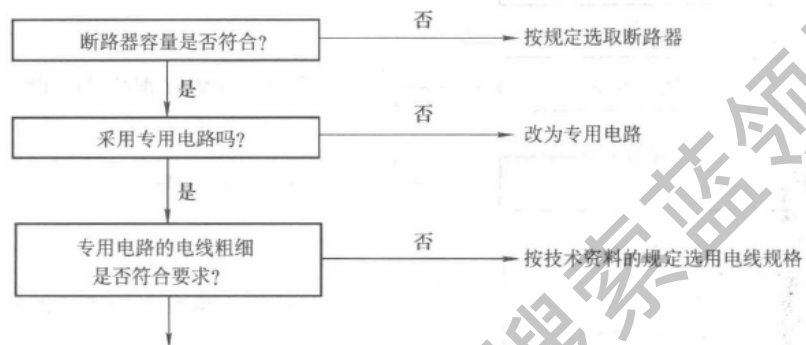
图 14-3 制冷运转中断路器跳闸排除方法
