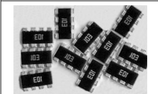
贴片排阻
