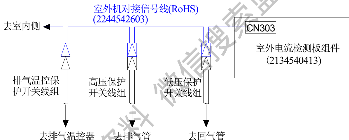
图七 保护器连接示意
