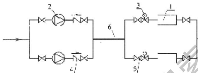
图5.2.8-3 循环泵和冷水机组之间共用集管连接方式和阀门配置
