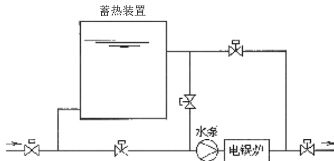
图7.4.9 串联的电水蓄热系统示意图
