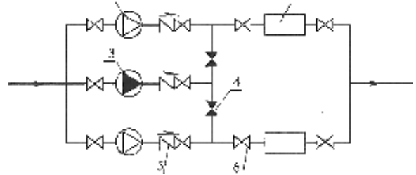
图5.2.8-2 循环泵和冷水机组之间一对一接管连接方式(设备用泵)和阀门配置
