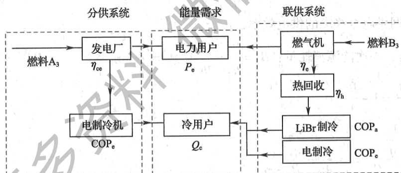
图10.4.3—3 联供、分产示意框图(三)
