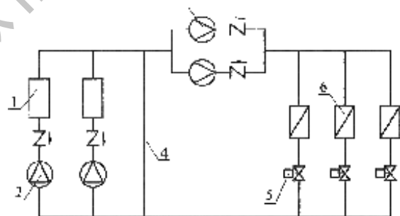
图5.2.9 空调冷水二次泵系统
