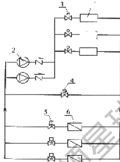
图5.2.10 空调冷水一次泵变流量系统
