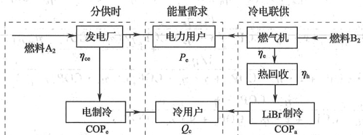
图10.4.3-2 联供、分产示意框图(二)
