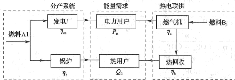
图10.4.3-1 联供、分产示意框图(一)
