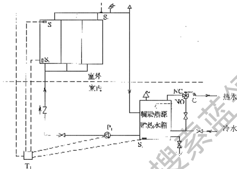
图9.3.4—1 直接系统温差循环控制系统图
