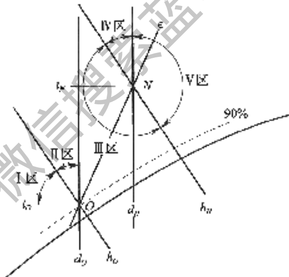
图 5.7.1-1 不同的夏季室外空气状态点在 h-d 图上的区域划分
