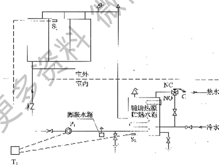
图9.3.4—2 间接系统温差循环控制系统图
