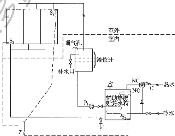
图9.3.6—2 排回系统
