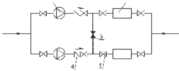
图5.2.8-1 循环泵和冷水机组之间一对一接管连接方式(无备用泵)和阀门配置
