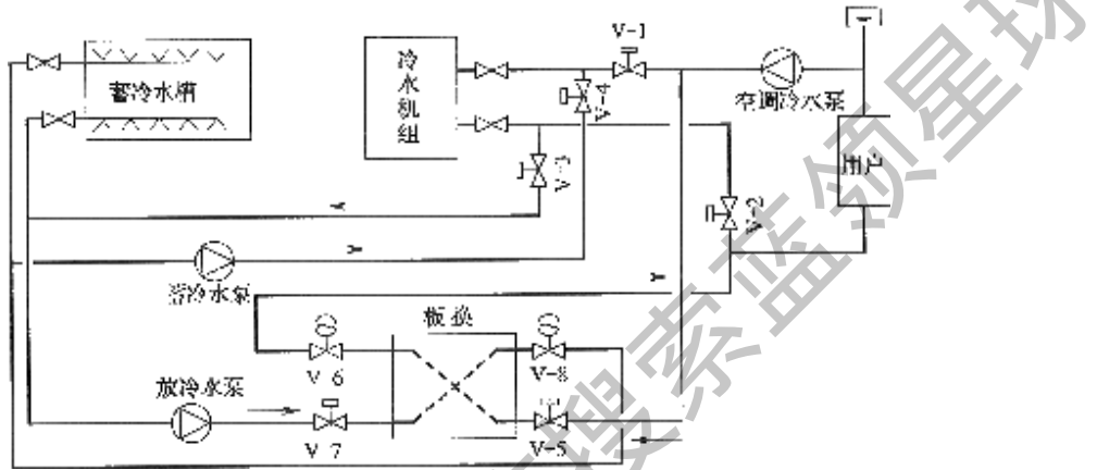
图7.3.8 并联方式水蓄冷系统
