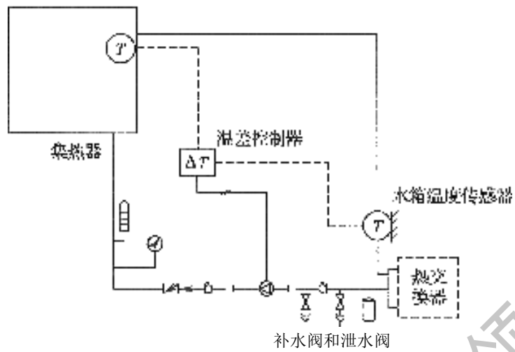
图9.3.6—3 防冻液系统
