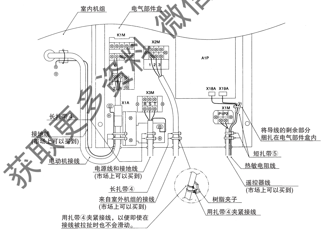
A向视图
