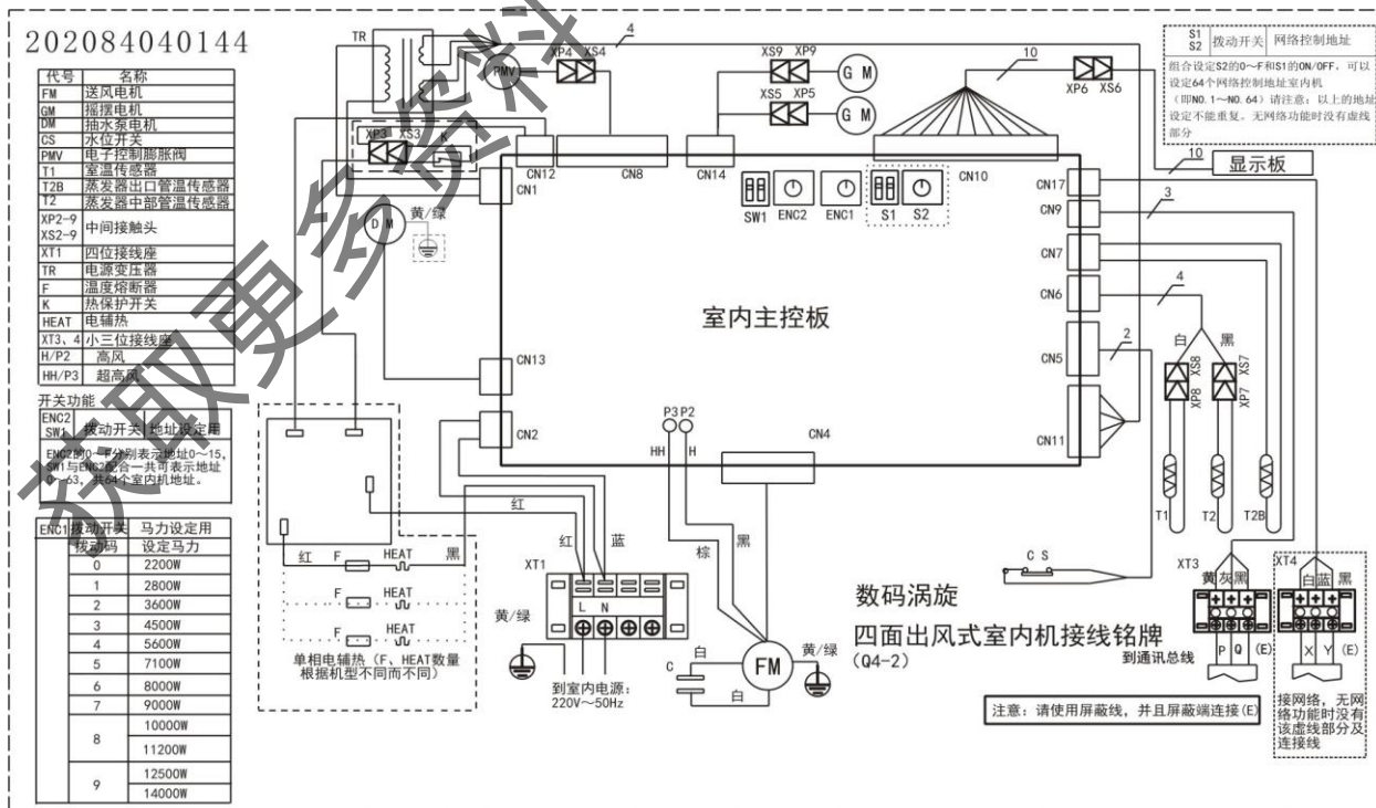
MDVH-J90Q4/DN 1 -C
