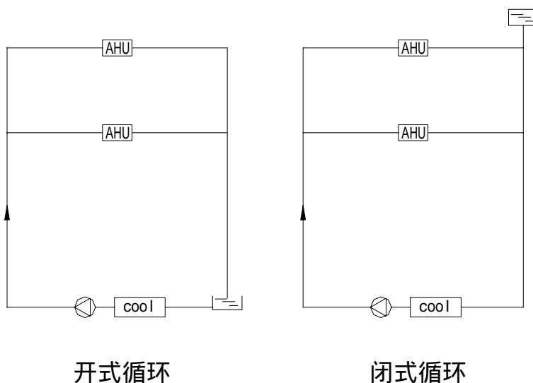
B-1 开式循环和闭式循环
