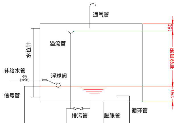
B-10 膨胀水箱
