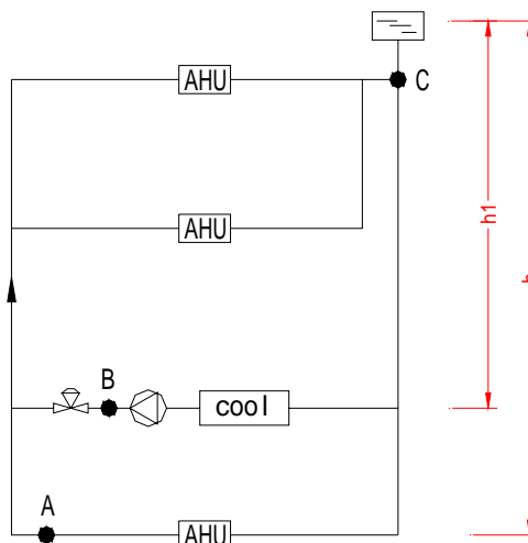
B-5 水系统的承压
