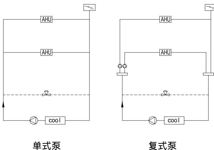
B-4 单式泵和复式泵
