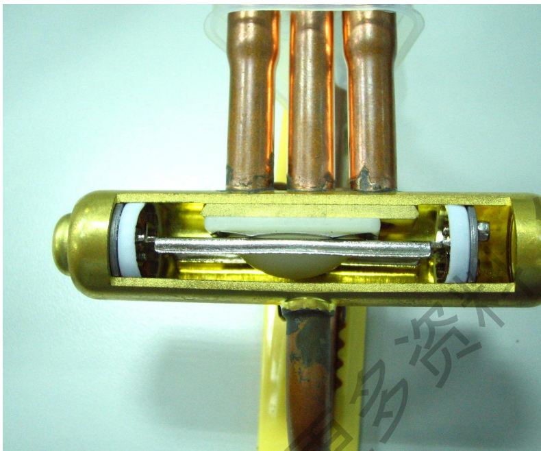
主阀体内部构造图
