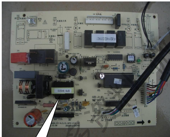
开关电源方案：变压器焊在PCB板上。
