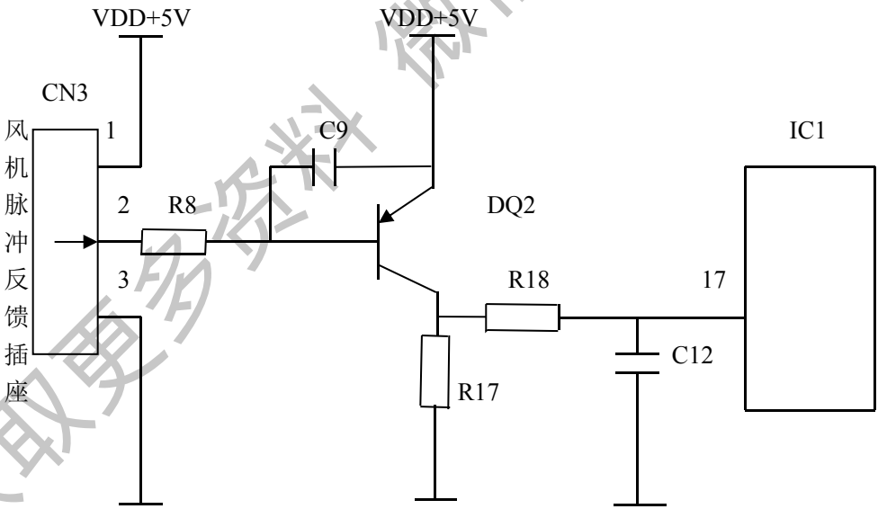
室内风机风速反馈电路如图 b
