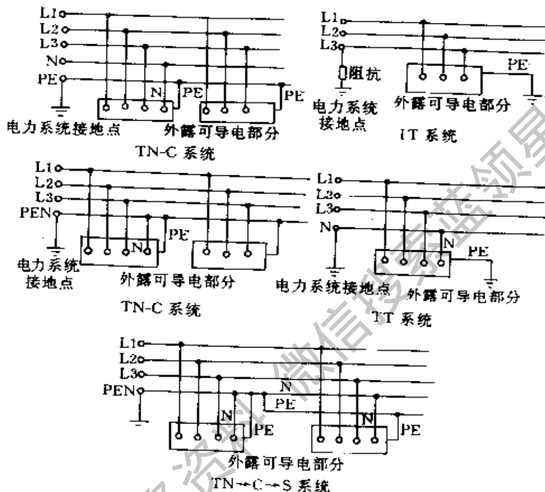
图24-1 按接地方式分类的电力系统
