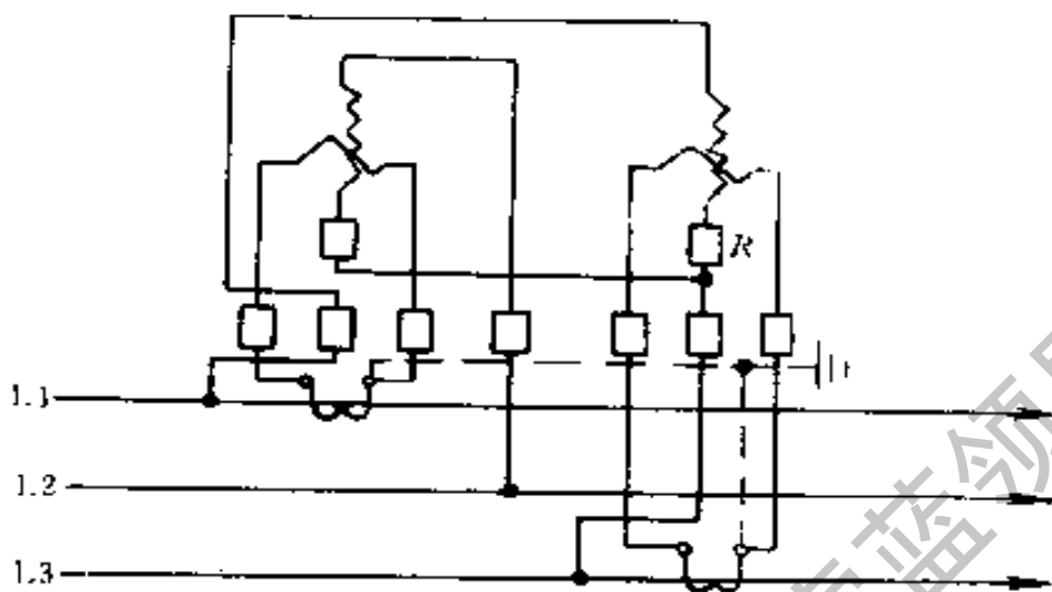
图 5-31 三相无功电度表经电流互感器的接线
