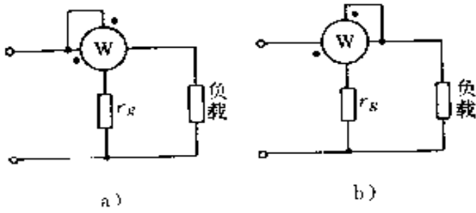
图 5-11 用功率表测量功率中的接线 如图 5-12 所示。
