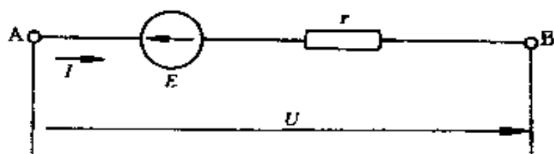
图 3 5 电能说明图
