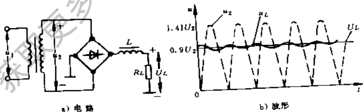
图 4-19 单相电感滤波桥式整流电路
