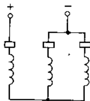
b) 两相并联与一相串联
