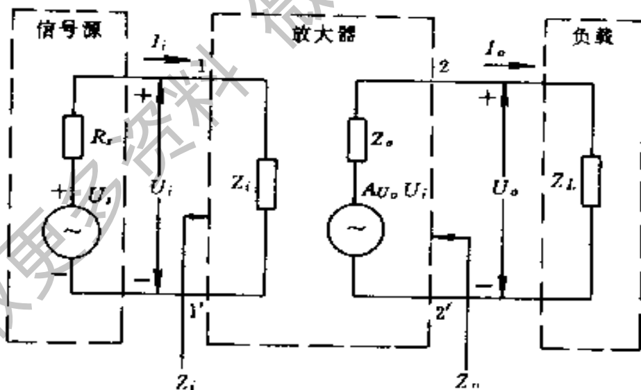
图 4.5 放大器的增益
