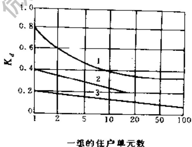
图 17-1 住宅群需要系数 K_d 值
