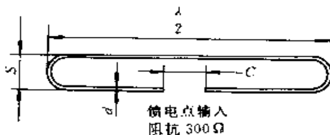
图23-3 折合振子天线
