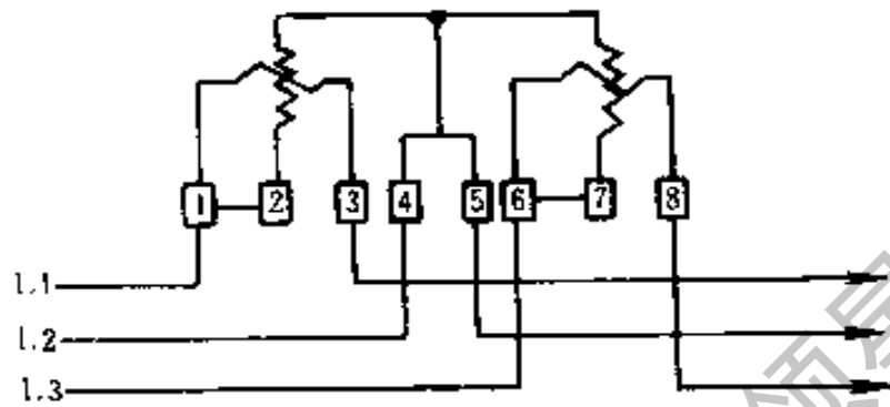
图 5-23 三相三线有功电度表直接接线
