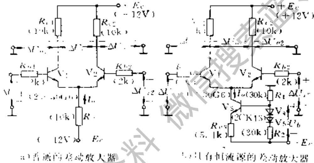
图 4-7 差动放大器
