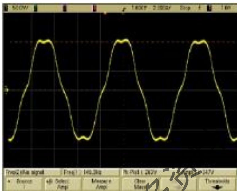
无刷直流电机驱动波形（方波）
