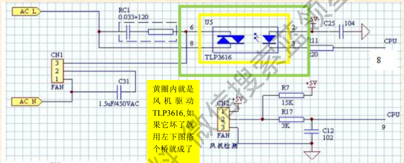
这是海信99系列挂机风机驱动和“霍尔”采样电路
