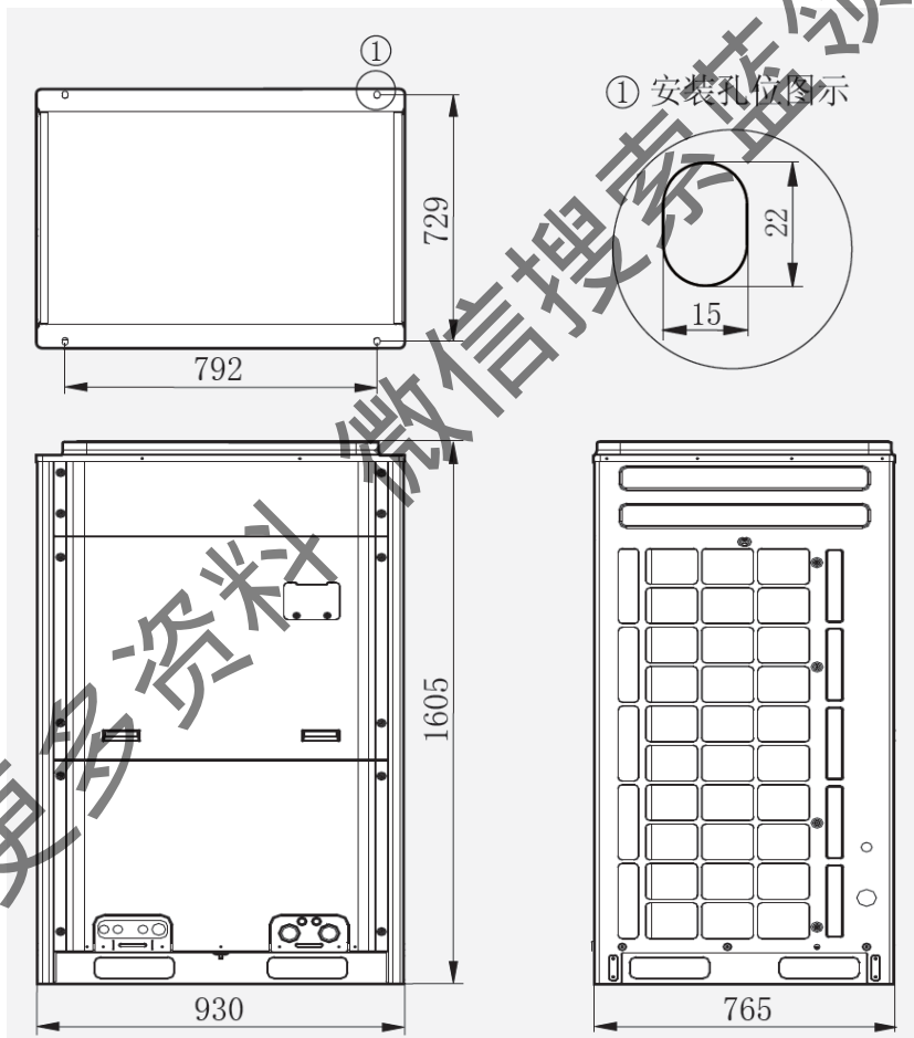
GMV-224~280WM/A 多联式空调机组安装 GMV-224~280WM/B
