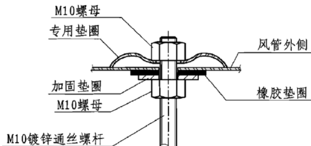
正压风管加固方式
