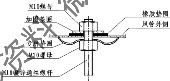
负压风管加固方式
