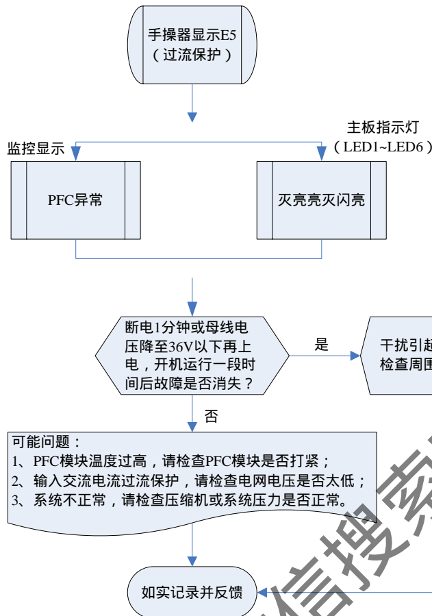
图 3.1.2.1 PFC 板异常故障检查流程图
