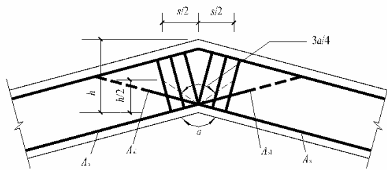
图 9.2.12 折梁内折角处的配筋
