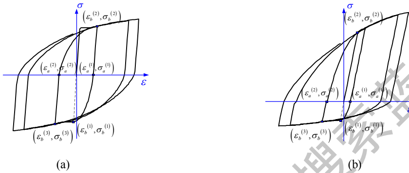
图 C.1.3 钢筋反复拉压应力-应变曲线
