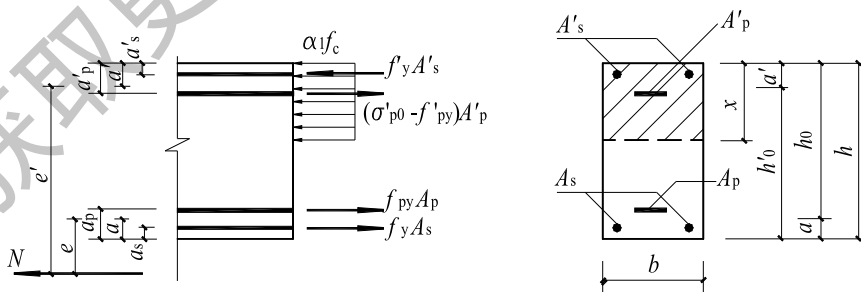
(a) 小偏心受拉构件
