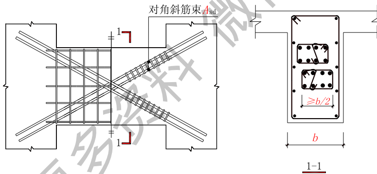
图 11.7.10-3 对角暗柱配筋连梁
