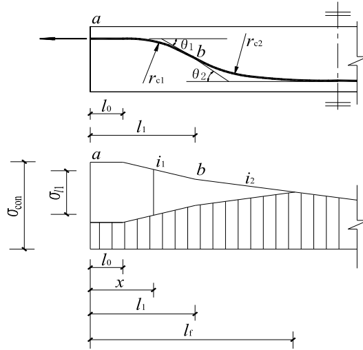
图 J.0.3-2 两条圆弧形曲线组成的预应力筋的预应力损失 \sigma_{II}
