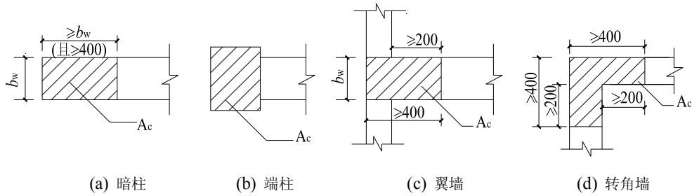
图 11.7.19 剪力墙的构造边缘构件
