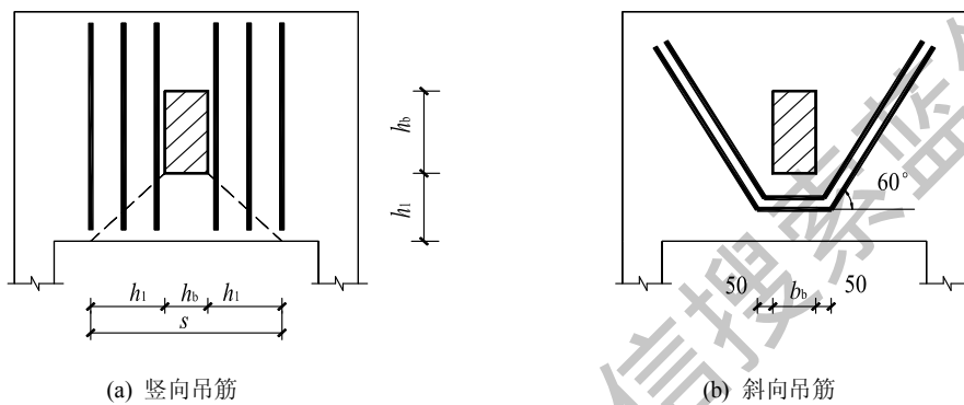
图 G.0.11 深梁承受集中荷载作用时的附加吊筋
