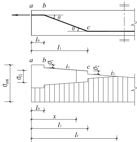
图 J.0.3-3 折线形预应力筋的预应力损失 \sigma_{II}
