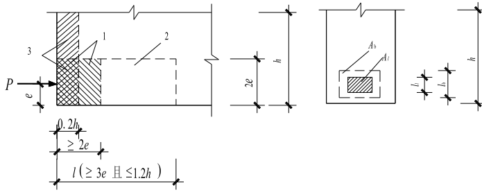
图 10.3.8 防止端面裂缝的配筋范围
