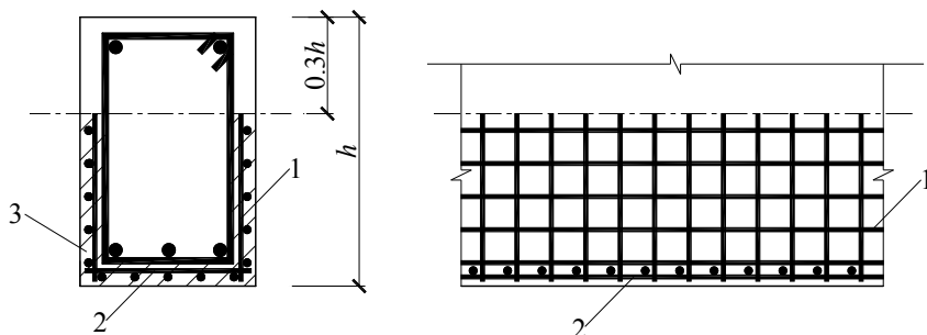
图 9.2.15 表层钢筋配置筋构造要求
