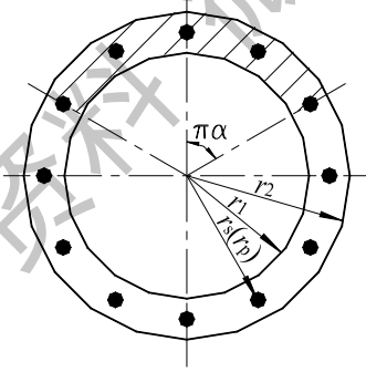
图 E.0.3 沿周边均匀配筋的环形截面
