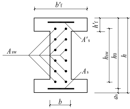
图 6.2.19 沿截面腹部均匀配筋的 I 形截面
