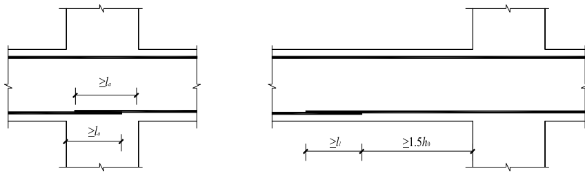
(a) 下部纵向钢筋在节点中直线锚固 (b) 下部纵向钢筋在节点或支座范围外的搭接
