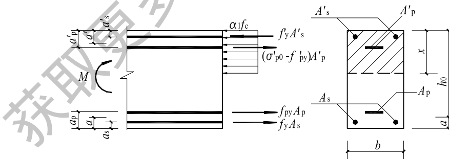
图 6.2.10 矩形截面受弯构件正截面受弯承载力计算
