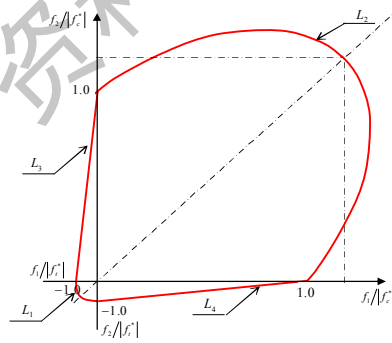
图 C.4.2 混凝土二轴应力的强度包络图
