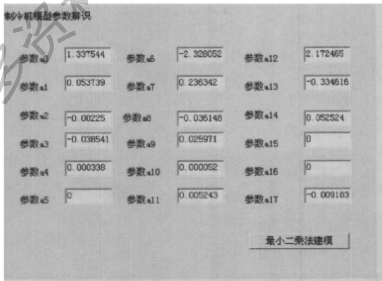
图 4.4 制冷机能耗模型系数
