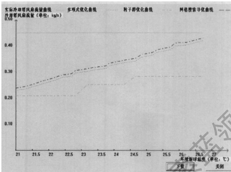
图 5.11 40%冷负荷, 冷冻水供水温度为7°C下冷却塔空气质量流量设定点的优化
