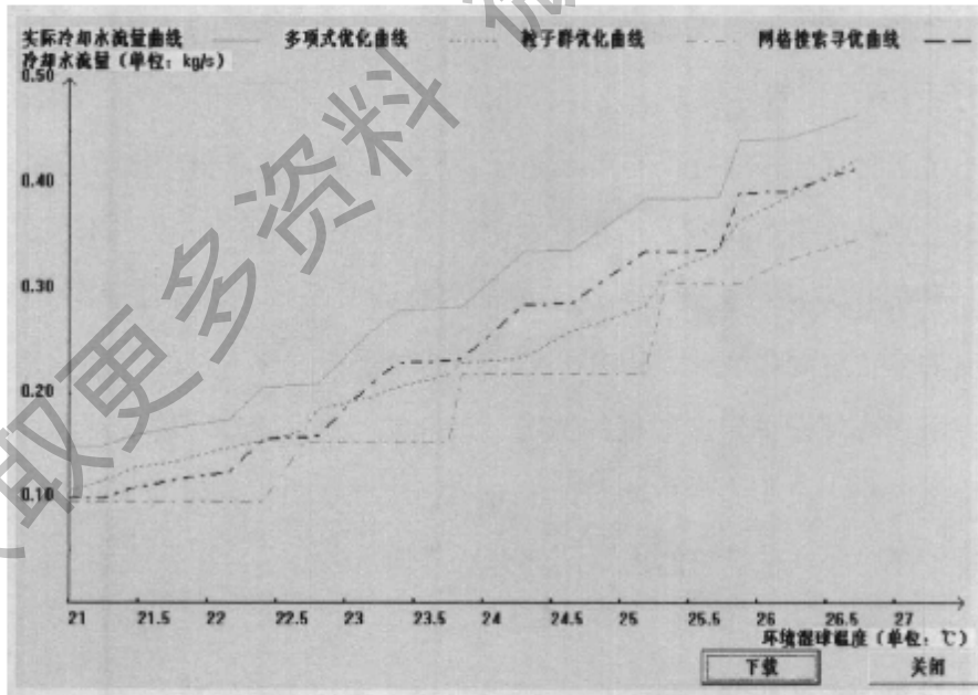
图 5.12 40%冷负荷, 冷冻水供水温度为7°C下冷却水质量流量设定点的优化
