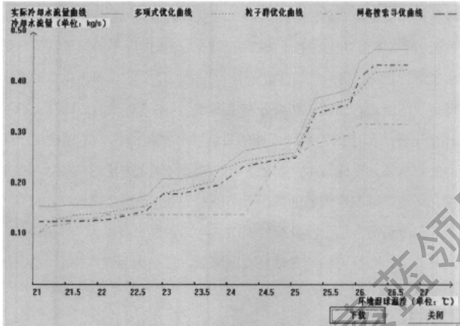
图 5.8 60%冷负荷，冷冻水供水温度为 9℃ 下冷却水质量流量设定点的优化
