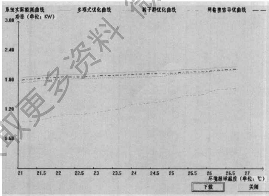
图 5.9 60%冷负荷，冷冻水供水温度为 9℃ 下空调制冷系统的能耗比较
