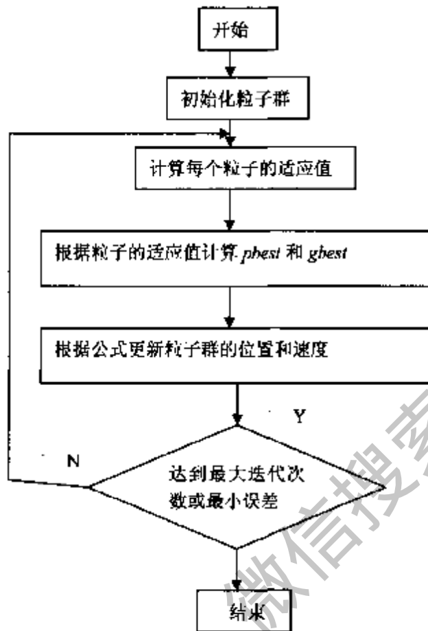
图 4.2 粒子群优化流程图
