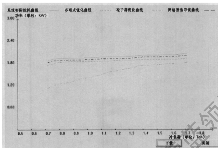
图 5.41 冷冻水供水温度为 7℃，环境湿球温度为 25℃下
