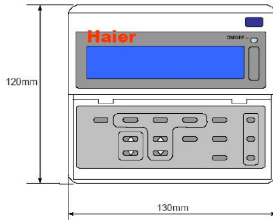
图一 打开反盖的示意图及外形尺寸
