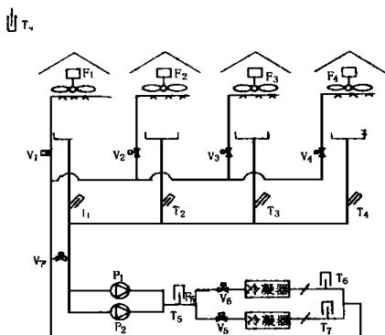
图 3-2 冷却水系统的测控点
