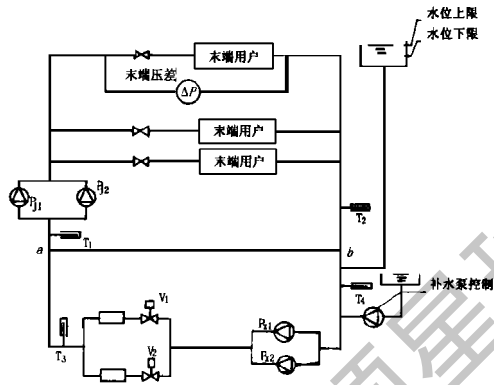
图 3-4 二级泵冷冻水系统
