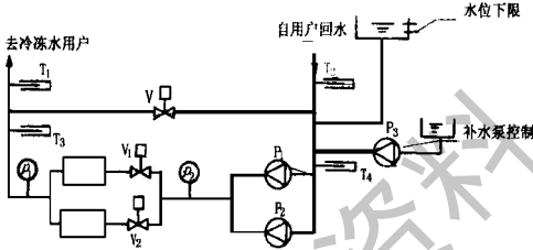
图 3-3 一级泵冷冻水系统
