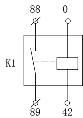
循环水泵控制
