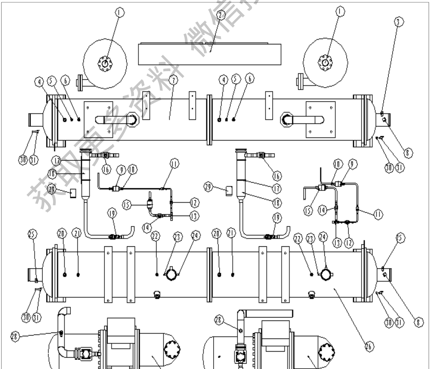
双机头满液式水冷螺杆机组爆炸图
