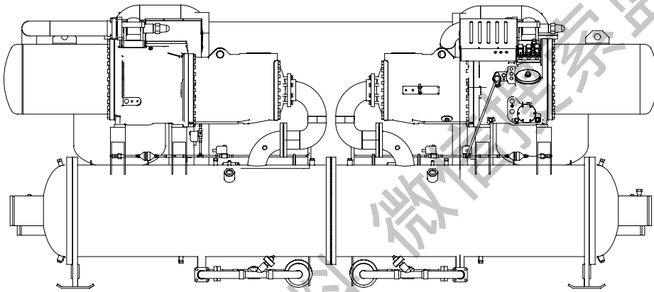
双机头满液式水冷螺杆机组外观图
