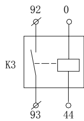
冷却塔风机控制
