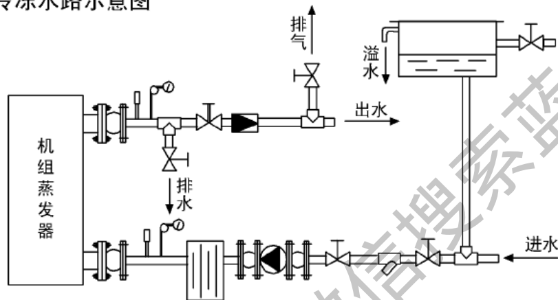
■ 冷冻水路示意图
