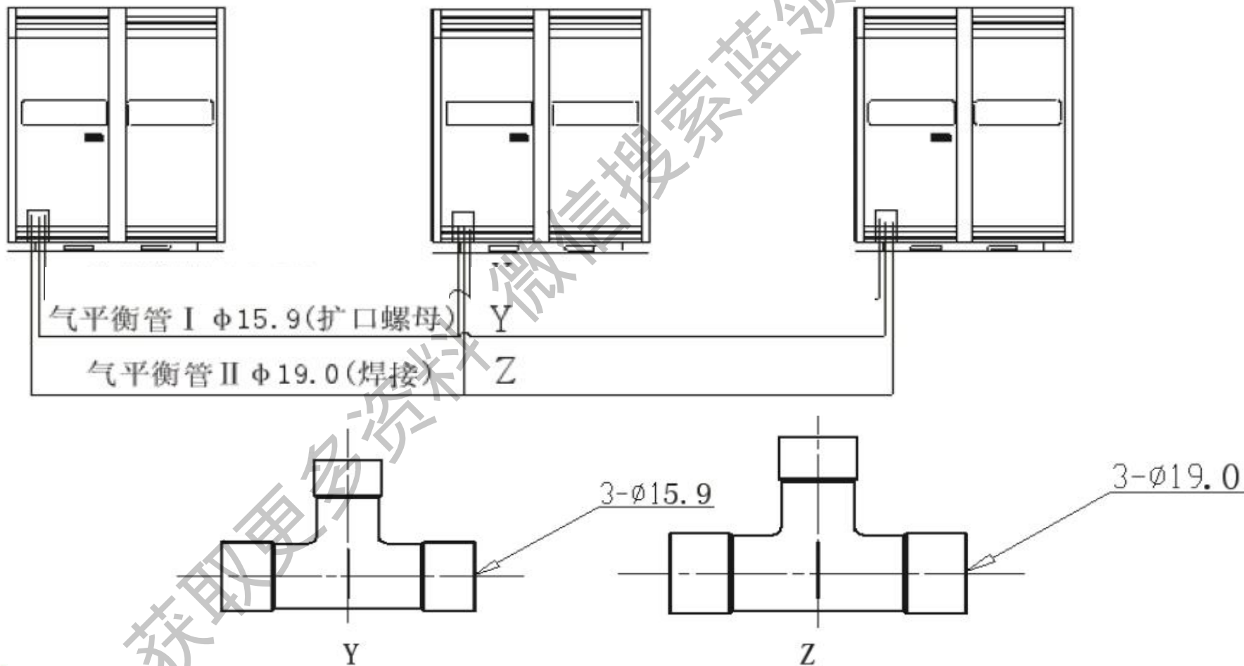
连接气平衡管的 T 型三通 Y, Z
