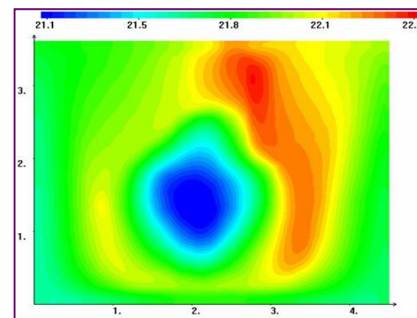
人员活动 区(1.5m) 温度场
