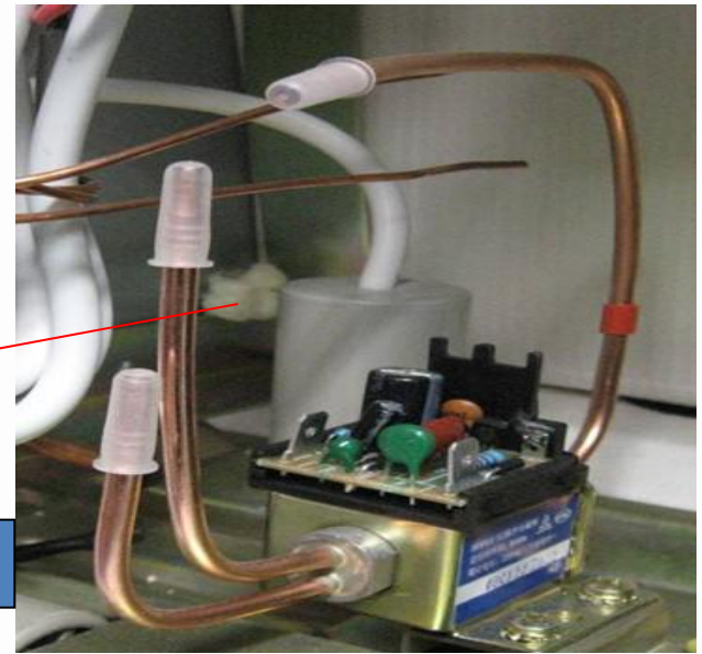
电磁阀
