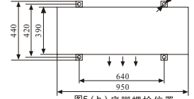
图5(b) 底脚螺栓位置
