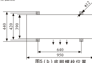
图5(b) 底脚螺栓位置
