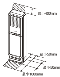
图1 操作空间
