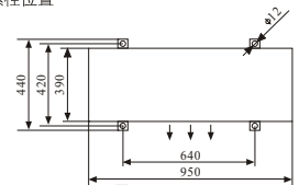
图5(b) 底脚螺栓位置
