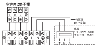
室外机端子排 KF-71LW/G(ZXF) KF-75LW/G(ZXF)
