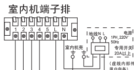
室外机端子排 KFRd-50LW/G(ZXF) KFRd-60LW/G(ZXF)
