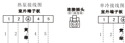
电源接线示意图
