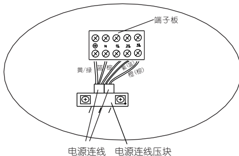
A. 冷暖机接线示意图
