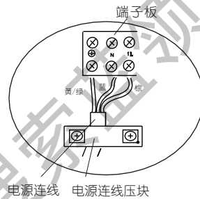
B. 单冷机接线示意图：
