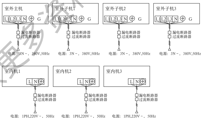
电源配线图
