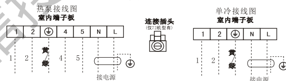
电源接线示意图
