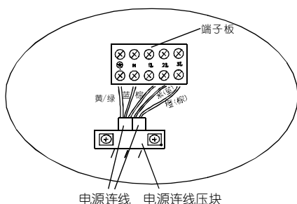
A. 冷暖机接线示意图
