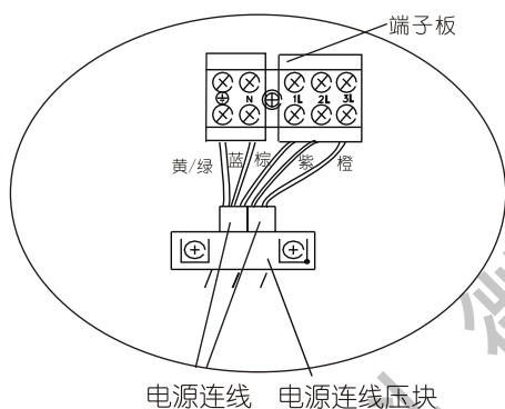
冷暖机室外机接线示意图
