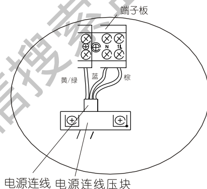
单冷机室外机接线示意图
