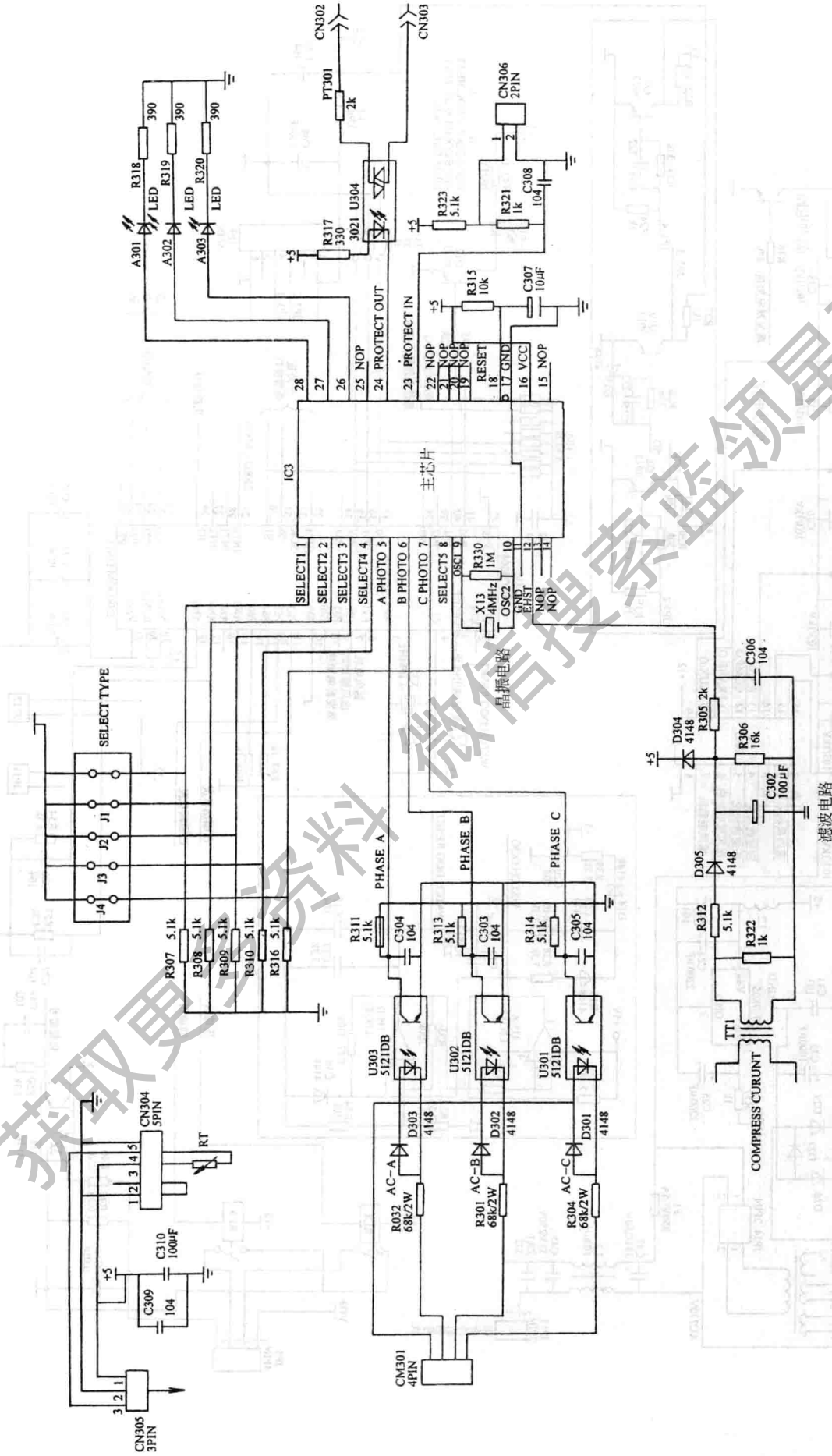
图 30 美的 KFR-75LW/ESD 柜式空调器室外机检测板控制电路图
