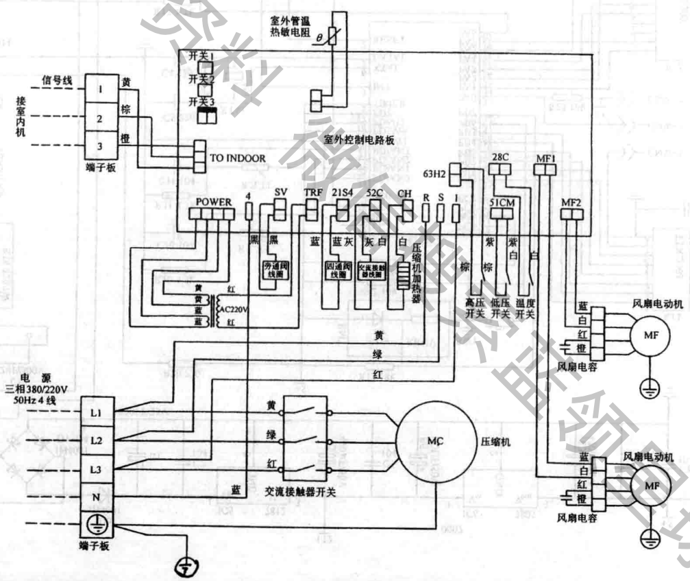
图 152 格兰仕 KFR-120LW/dSA 柜式空调器室外机控制电路图
