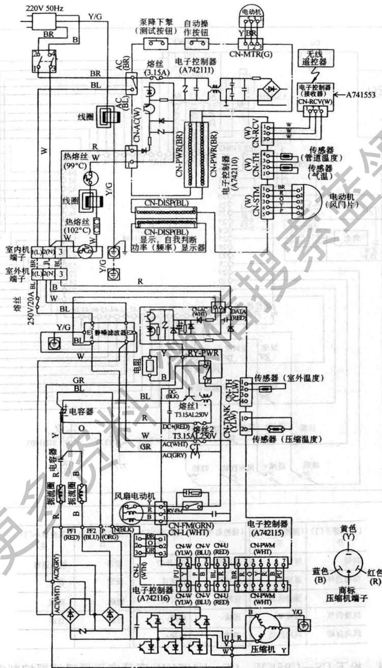
图 25 松下 CS—K105KW 变频空调器控制电路图
