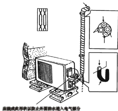
应做成此形状以防止外面的水进入电气部分
