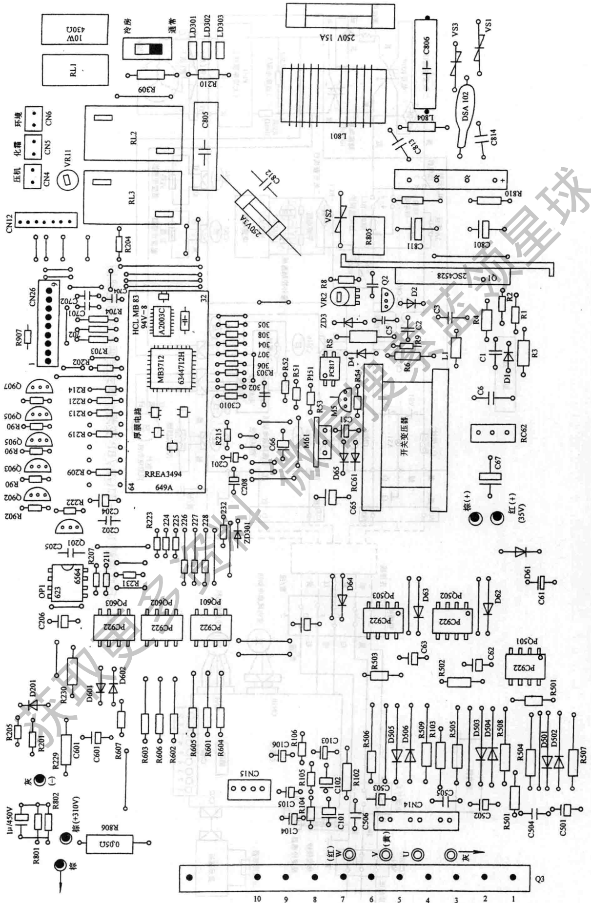
图 134 日立凉霸 KFR—36GW/BP 变频分体式空调器室外机元器件布置图
