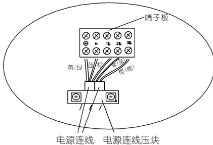
A. 冷暖机接线示意图
