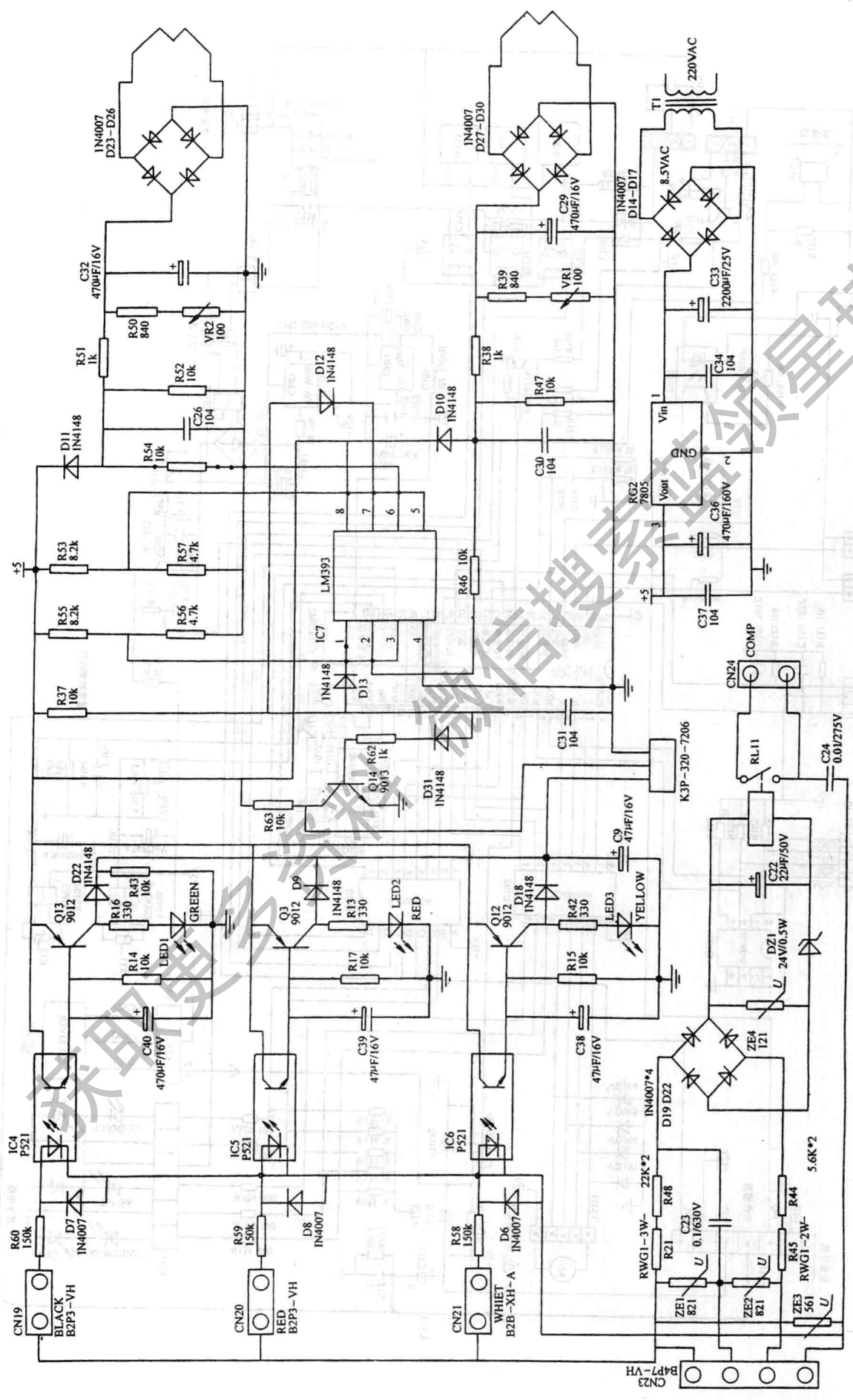
图 77 海信 KFR—7206LW/D 柜式空调器室外机微电脑控制电路图
